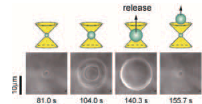
レーザー光の周りで観測された、有機溶媒の生成・消滅振動
