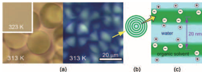
(a)水と3-メチルピリジンの混合溶媒に拮抗的な塩であるNaBPh 4 (Na + は親水性、BPh 4 - は疎水性)を加えた系での顕微鏡像。左は通常の透過光、右は同じ場所をクロスニコルの条件で撮影している (b)顕微鏡像から示唆された多重ベシクル構造の模式図(c)有機溶媒(3-メチルピリジン)が作るベシクル膜の描像
