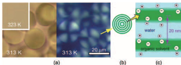
(a)水と3-メチルピリジンの混合溶媒に拮抗的な塩であるNaBPh 4 (Na + は親水性、BPh 4 - は疎水性)を加えた系での顕微鏡像。左は通常の透過光、右は同じ場所をクロスニコルの条件で撮影している。(b)顕微鏡像から示唆された多重ベシクル構造の模式図(c)有機溶媒(3-メチルピリジン)が作るベシクル膜の顕微鏡像
